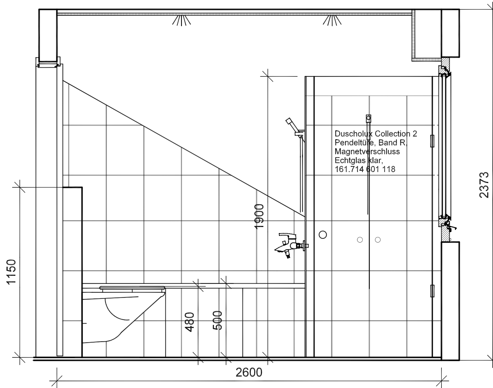
Ansicht B
