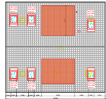
Dachdraufsicht
