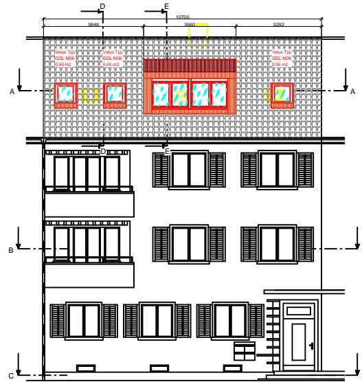
Ansicht Töstalstrasse
