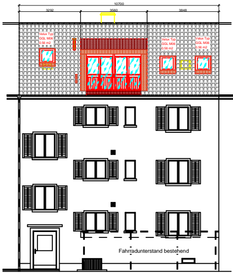
Ansicht Hinterhof
