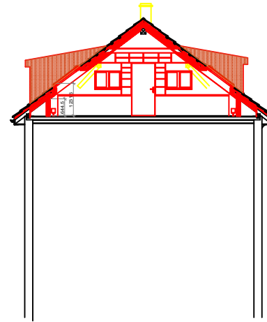
Schnitt D-D Dachstock Bürobereich
