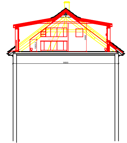
Schnitt E-E Dachstock Sitzungsraumbereich
